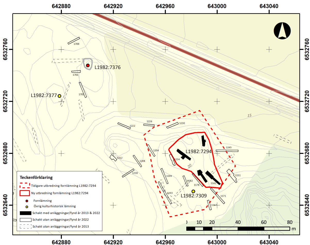
Figur 7. Schaktplan över fornlämning L1982:7294 och L1982:7376. Skala 1: 2000. © Lantmäteriet Dnr R50367921_150001.
