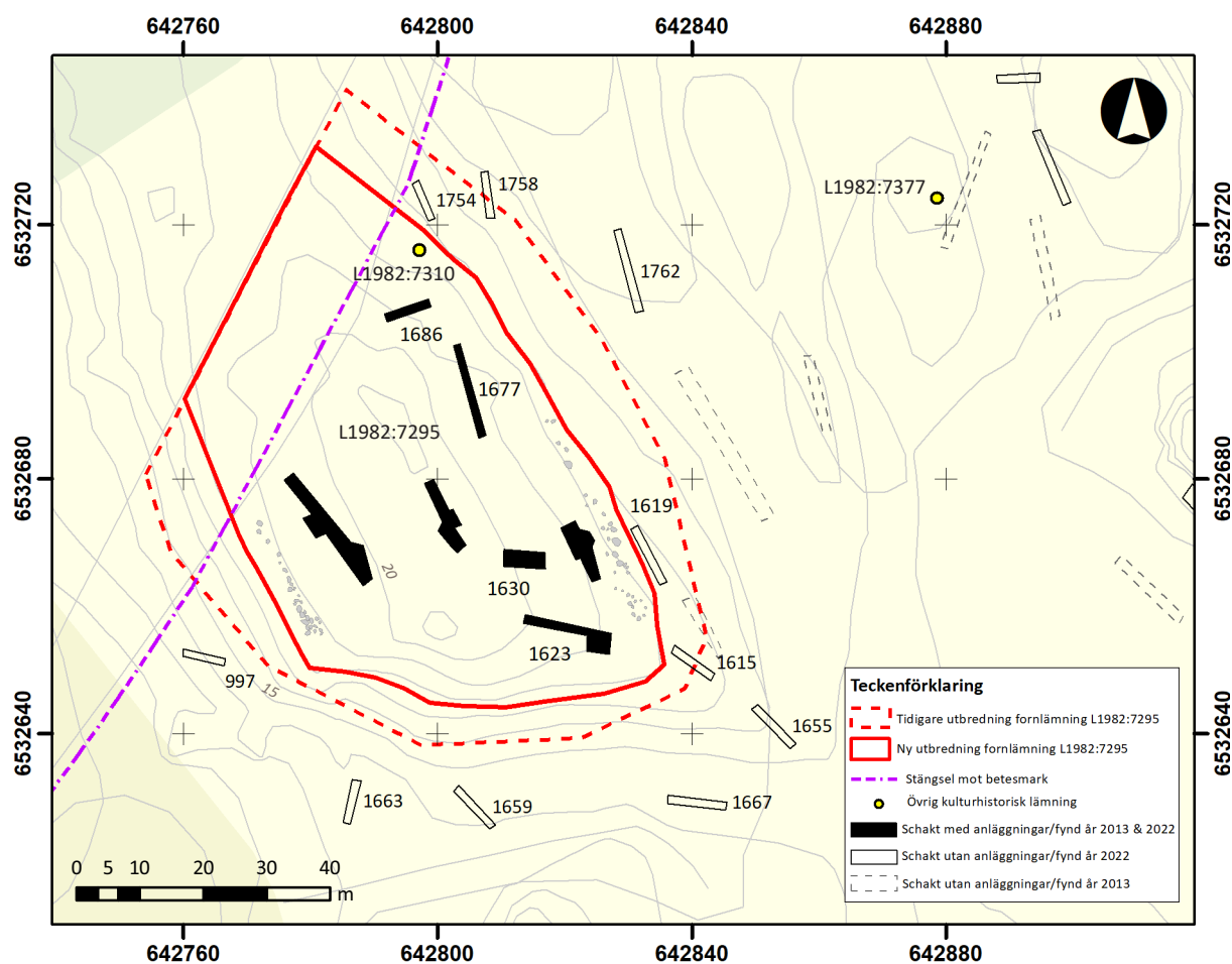
Figur 8. Schaktplan över fornlämning L1982:7295. Skala 1: 1200, © Lantmäteriet Dnr R50367921 150001.
