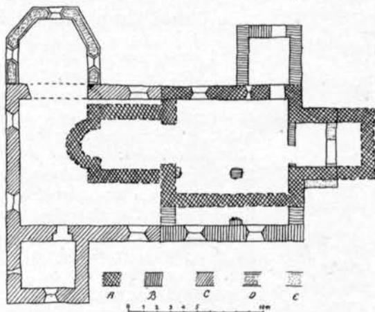
Fig. 62. Plan över Ö. Skrukeby kyrka.
